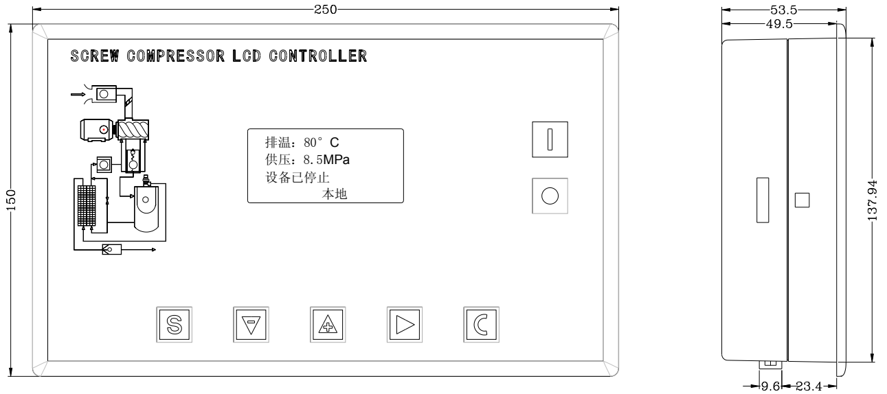
图 7、外围尺寸
