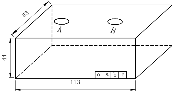
图 2、CT1 结构尺寸（ \phi 36 穿孔）
